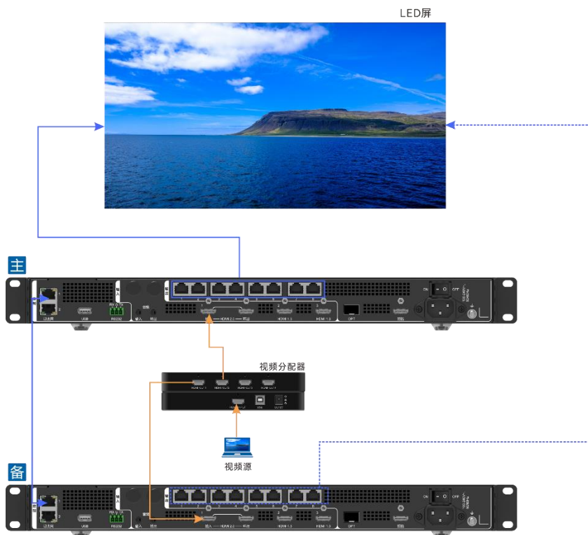
图 6-12 设备热备份连接图
