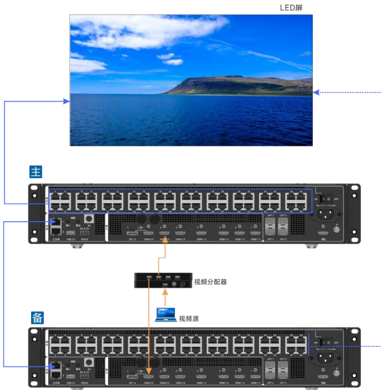
图 6-12 设备热备份连接图
