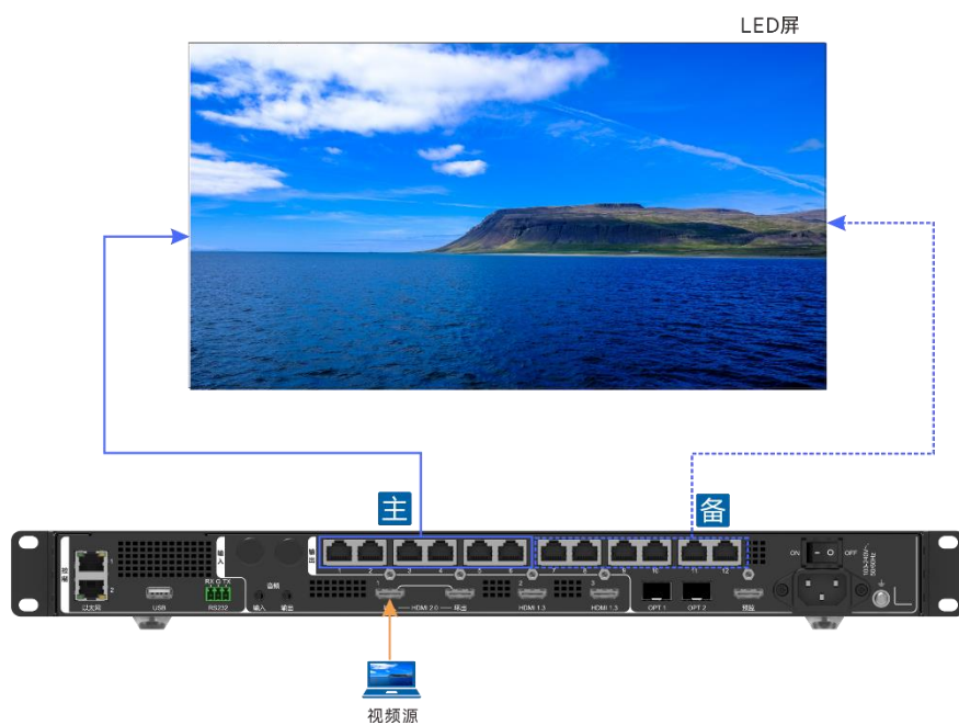
图 6-13 网口备份连接图
