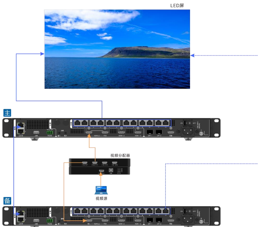
图 6-12 设备热备份连接图
