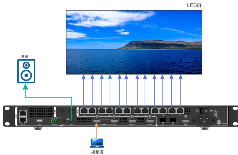
图 6-23 音频输出连接（音频输出接口连接）
