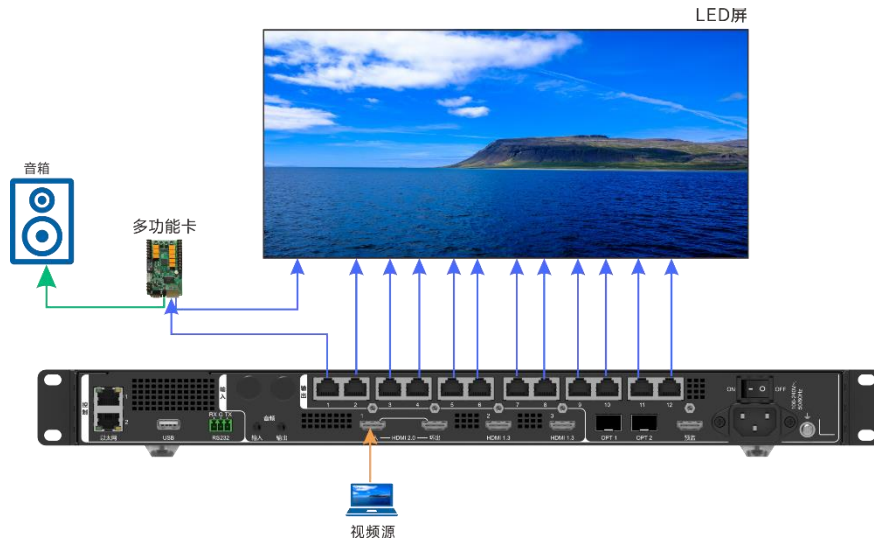
图 6-22 音频输出连接（多功能卡连接）
