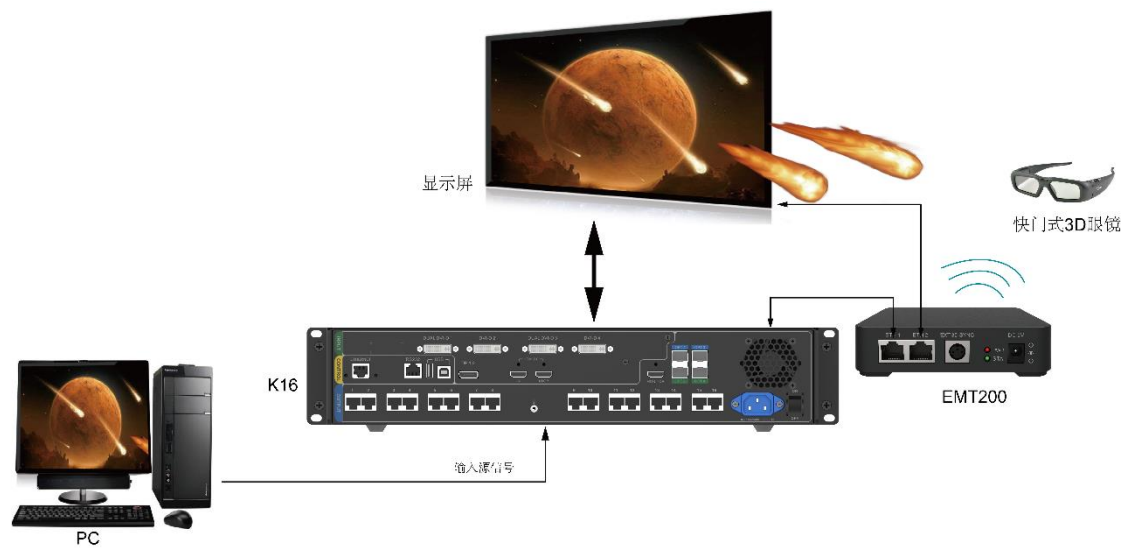
图5-28 硬件连接图
