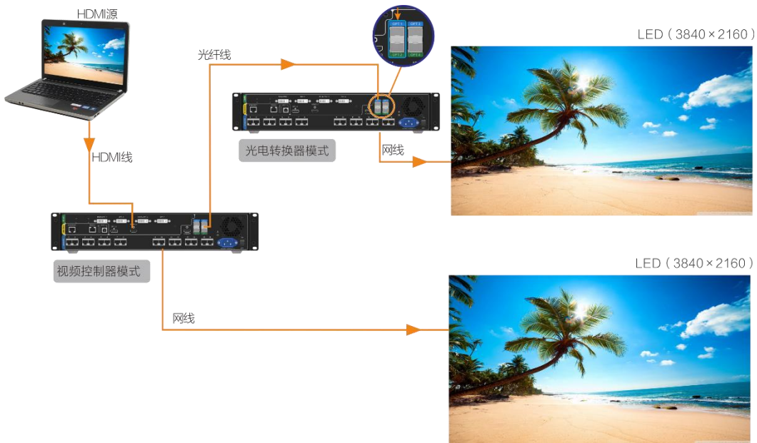
图5-25 光口复制连接图
