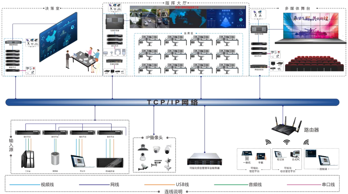
图3-3 典型组网-分布式和拼接器集中控制
