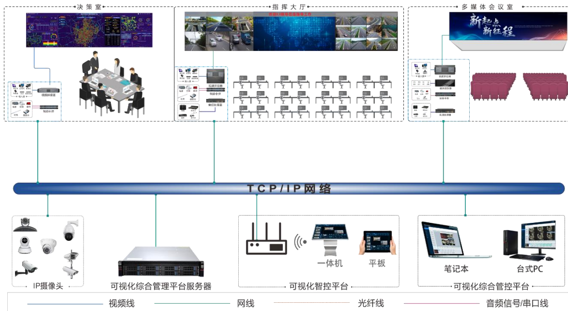
图3-1 典型组网-拼接器控制
