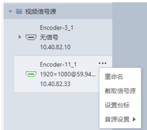
图3-51 输入源菜单
