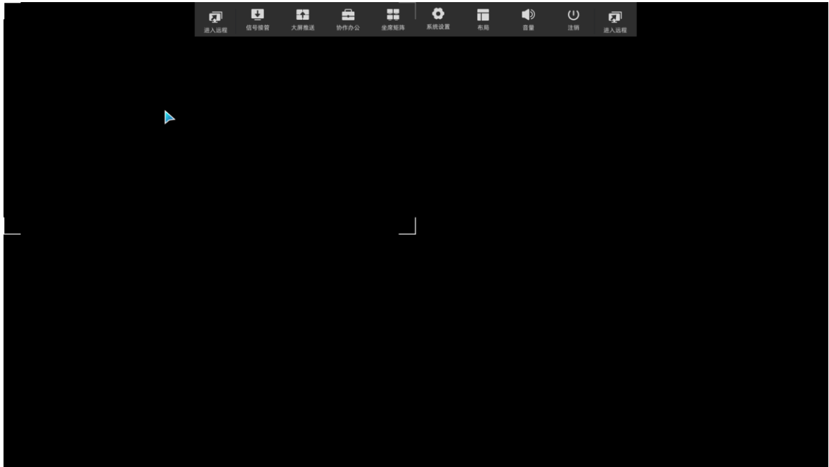
图4-2 坐席界面
