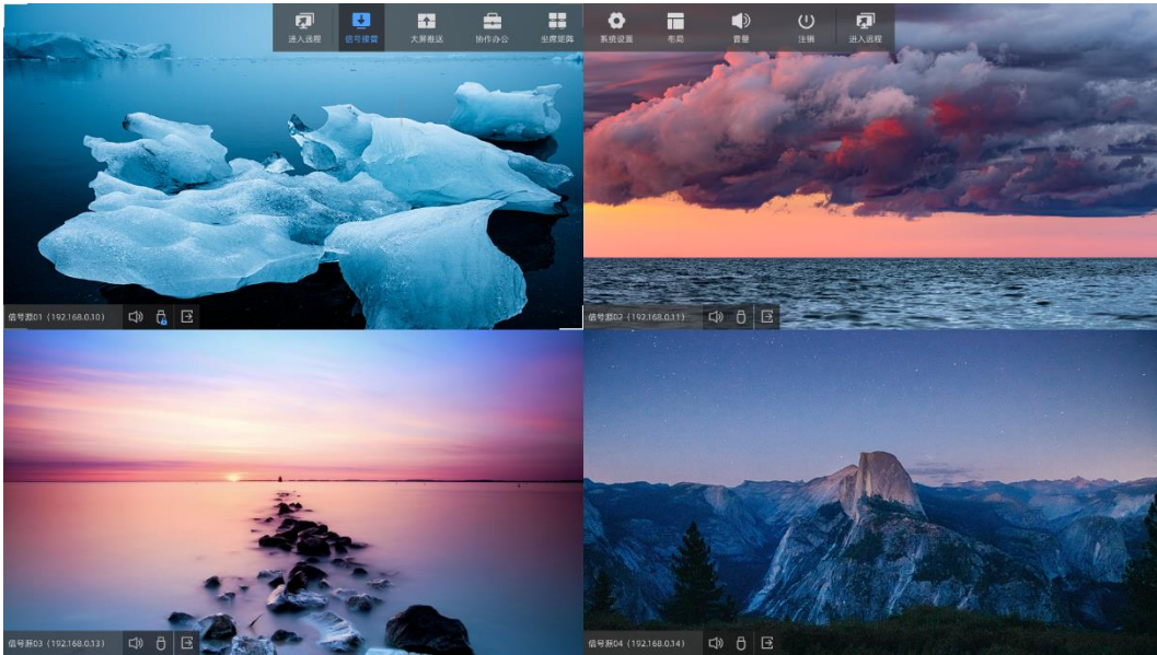
图4-13 U 盘挂载
