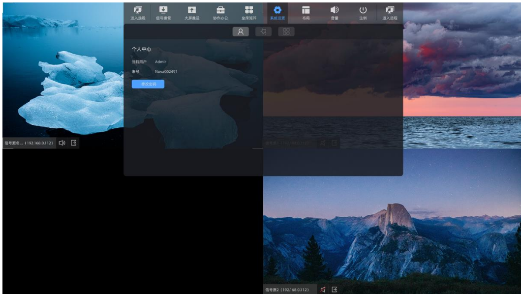
图4-15 系统设置
