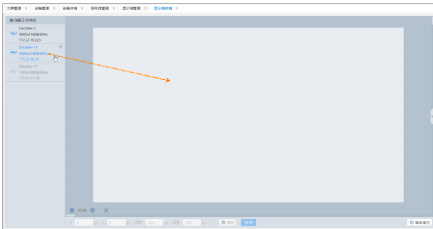
图3-9 显示墙配置
