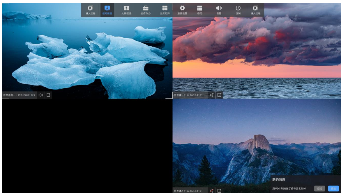
图4-10 推送请求
