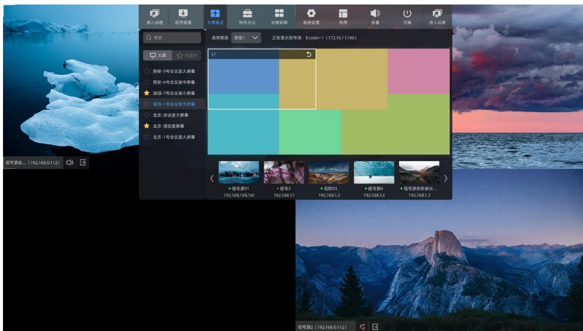
图4-11 大屏推送
