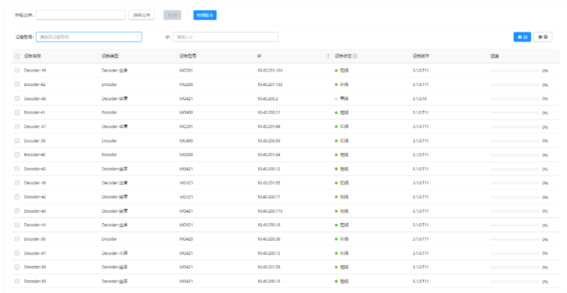
图3-34 固件升级
