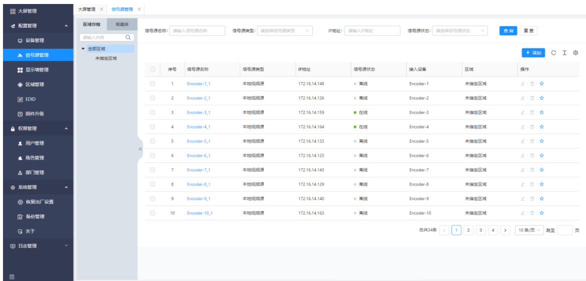
图3-25 信号源管理
