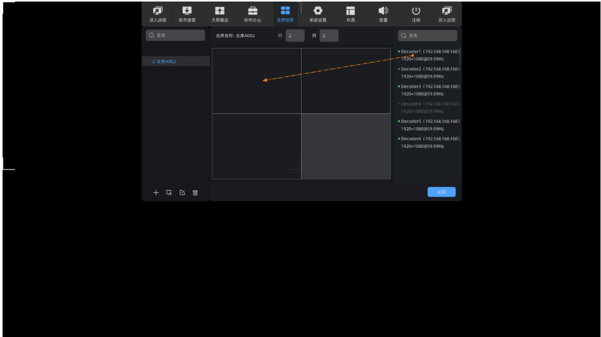
图4-4 坐席矩阵
