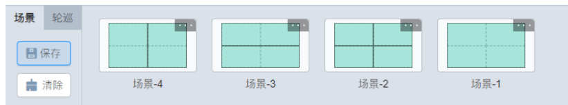
图3-46 场景列表
