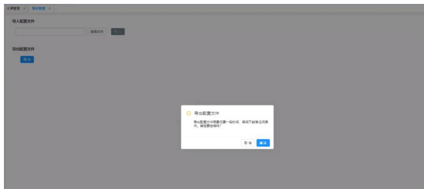
图3-65 备份导出
