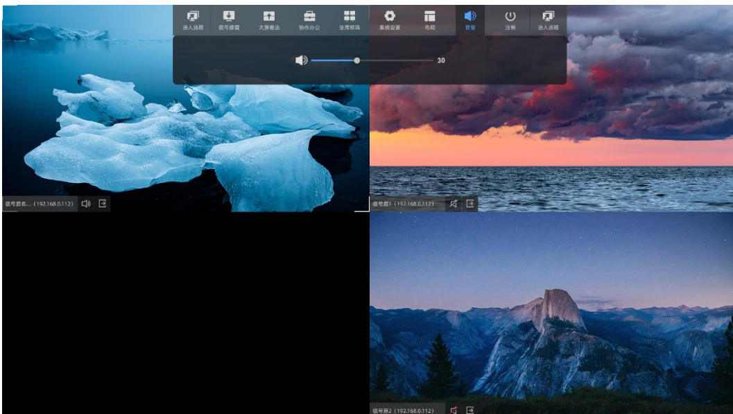
图4-14 音量
