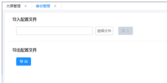
图3-64 备份管理
