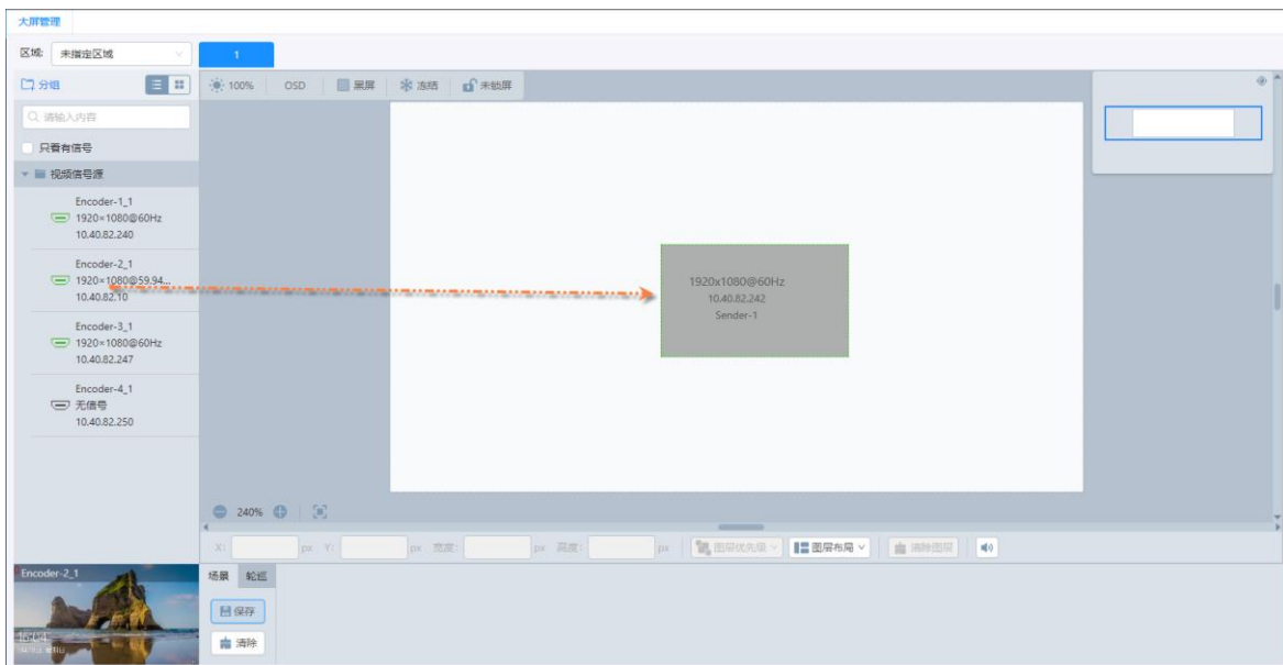
图3-37 添加图层
