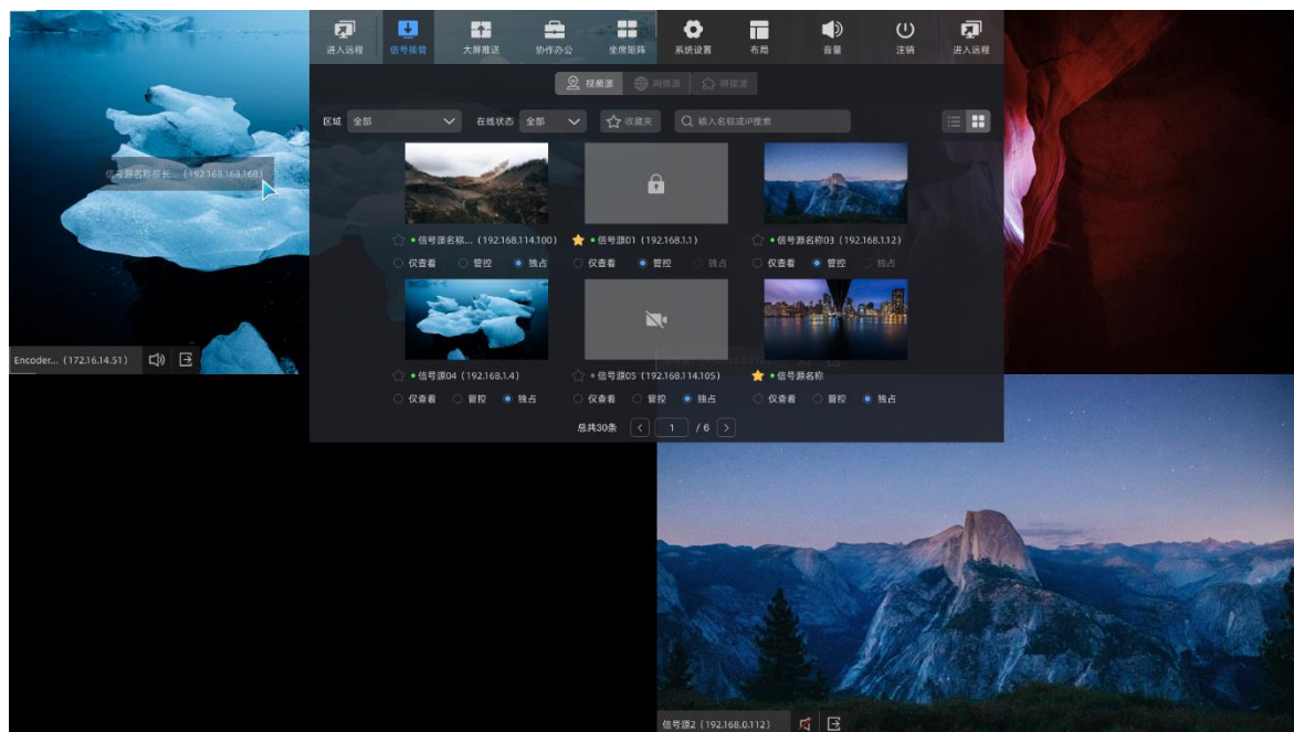
图4-7 信号源接管
