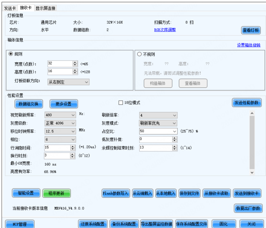
图5-34 接收卡
