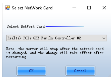
图13-3 选择网卡
