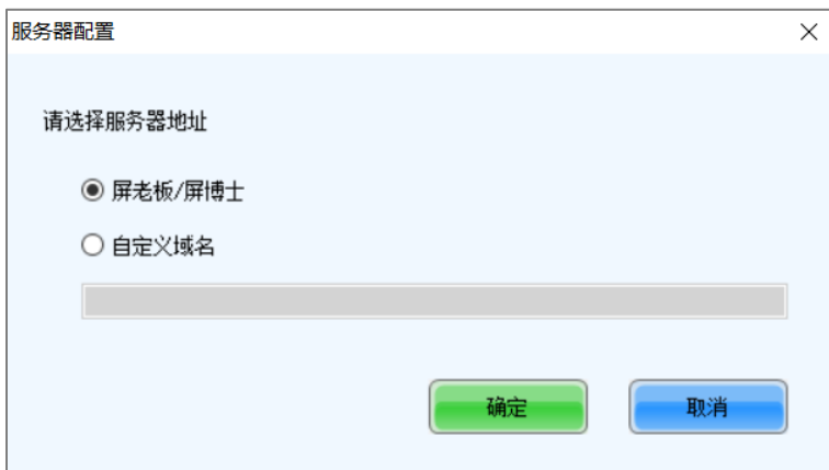
图11-4 服务器配置
