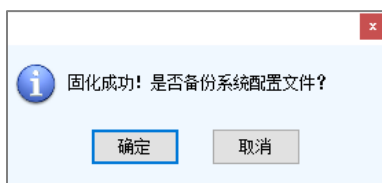
图5-32 固化成功
