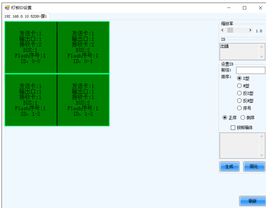
图8-8 设置灯板 ID (常规屏)
