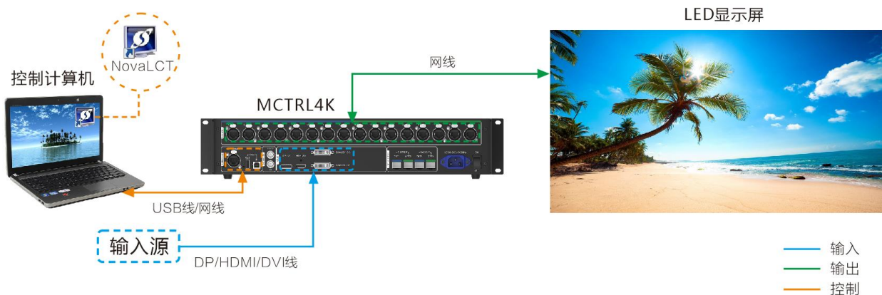
图3-1 硬件连接示例
