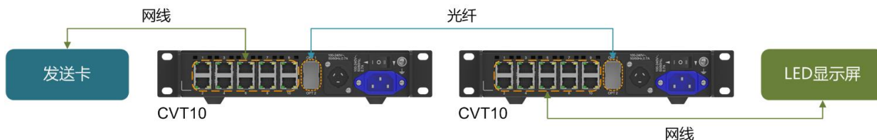
图8-22 两台 CVT10 的光电转换
