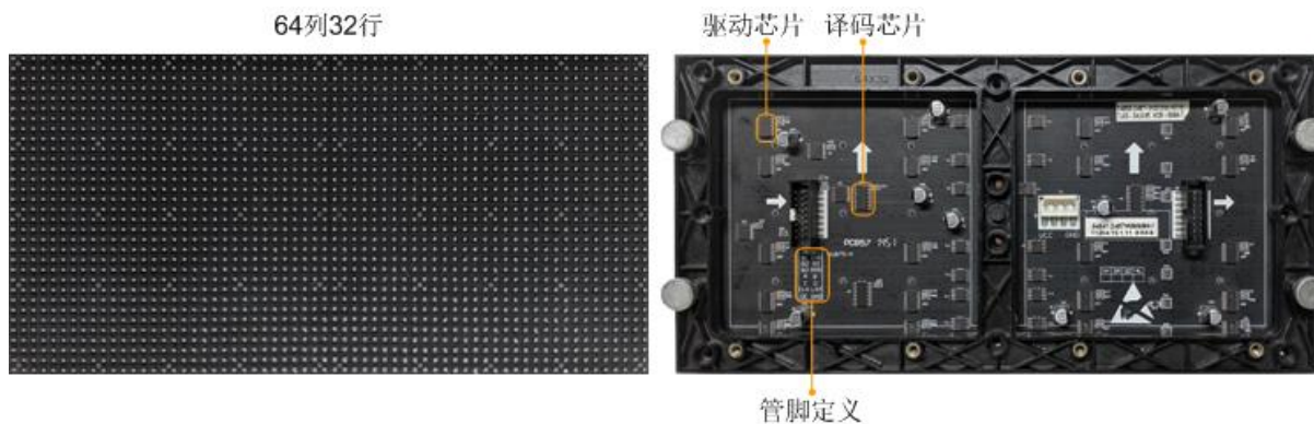
图5-5 灯板示例
