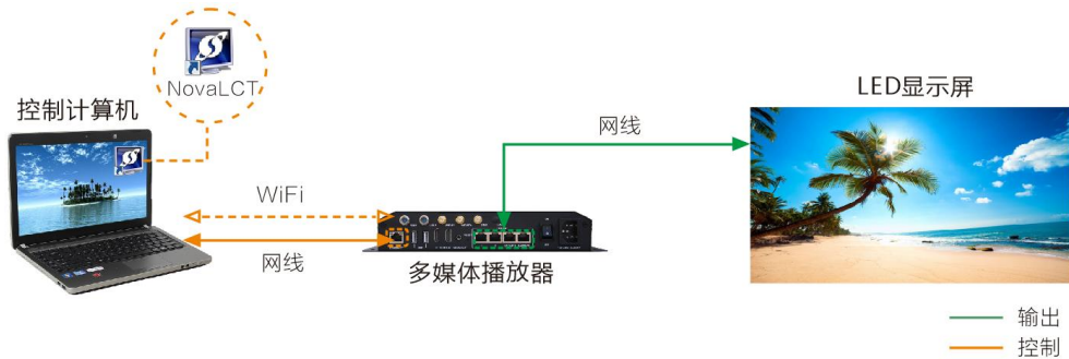
图3-1 直连
