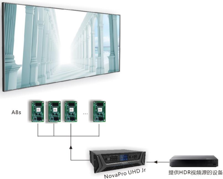
图5-22 HDR 系统架构图
