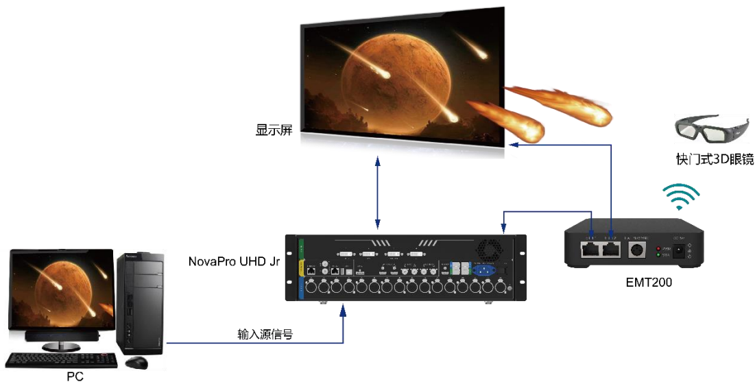
图5-28 硬件连接图
