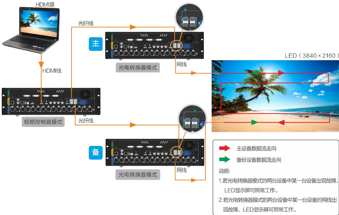
图5-24 光口热备份连接图
