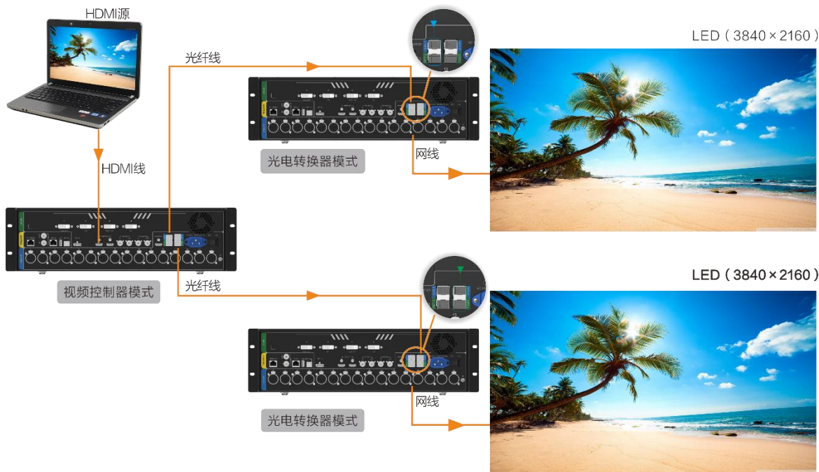
图5-25 光口复制连接图
